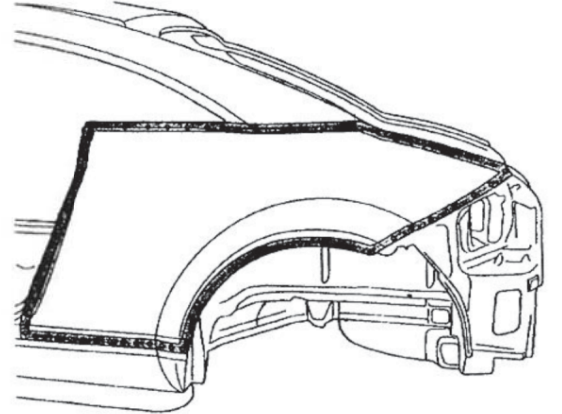
Audi TT mit Schweißfolge
